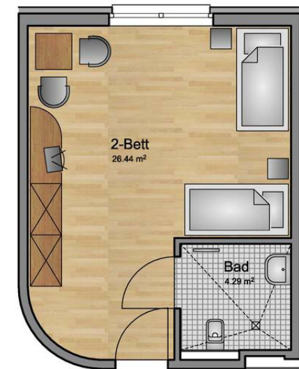
Doppelzimmer
